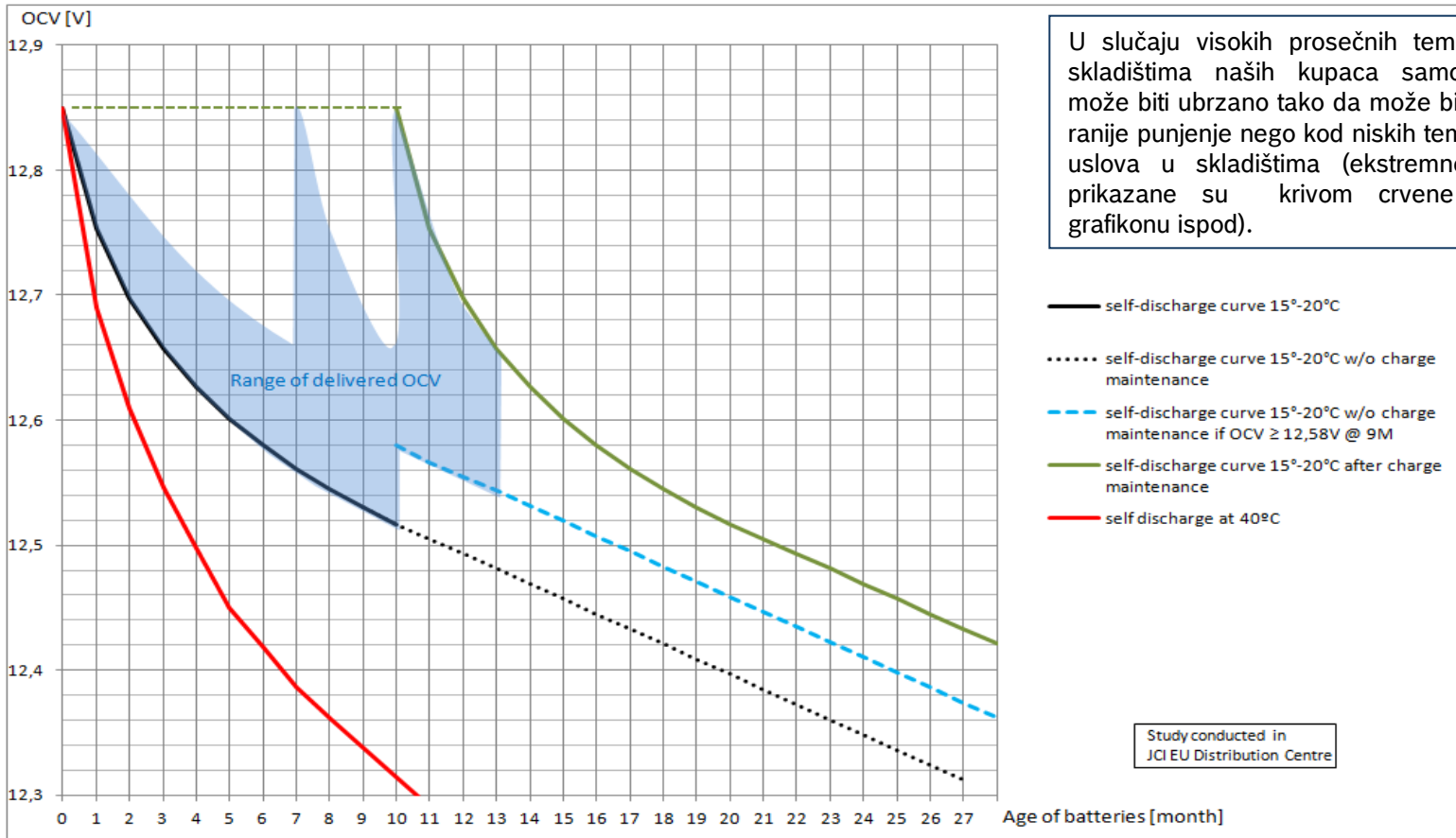
Dijagram kriva samopražnjenja (Normalna prosečna temperatura 15°C-20°C ; Za toplu klimu ispod 40°C crvena kriva)
