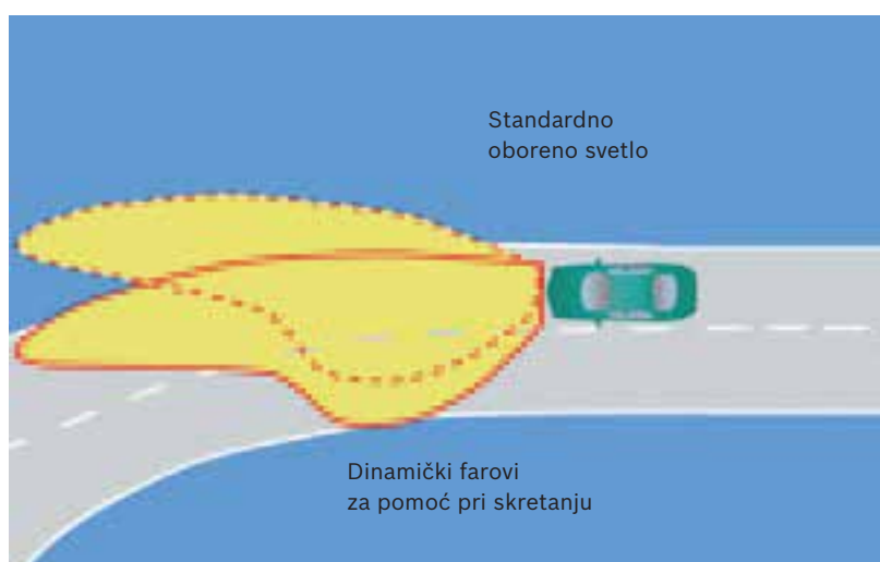
Osvetljavanje puta sa dinamičkim farovima za pomoć pri skretanju
