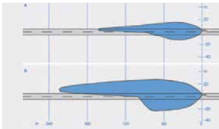
Poređenje: distribucija svetla kod halogene sijalice (gore) i distribucija svetla kod Xenon sijalice (dole)
